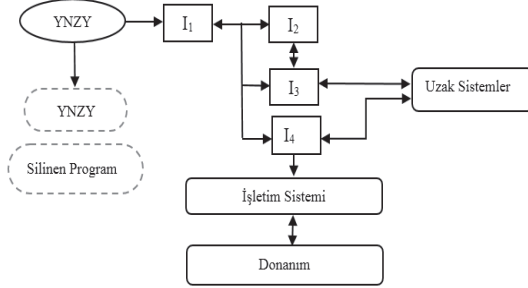
Şekil 2: Yeni nesil kötü amaçlı yazılımın blog diyagramı. 14
